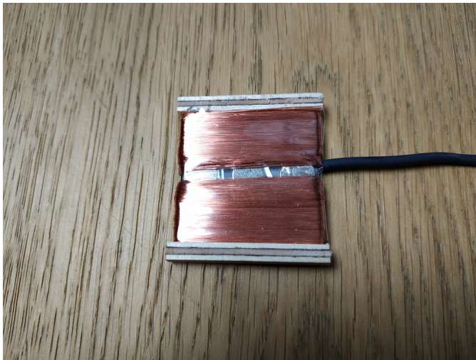
Alpen 3-String Humbucker mit hochpermeablem Silizium Kern
